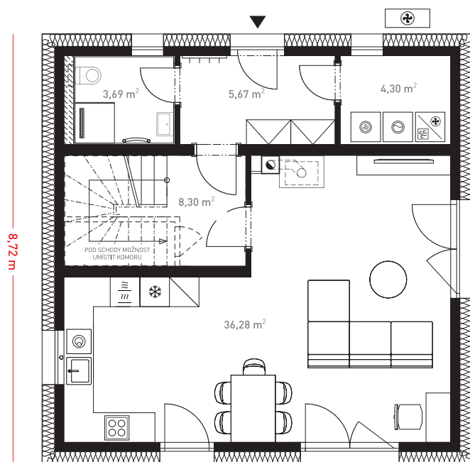
Přízemí
